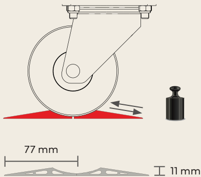
Kombination hoch – hoch
