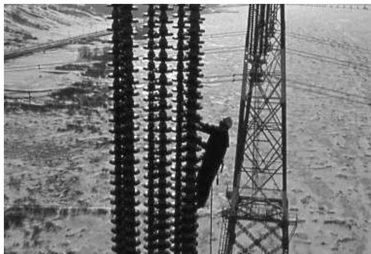
Inspection finale par Michel Bornais d'un ensemble d'isolateurs de suspension dans un pylône de la traversée 735KV du fleuve Saint-Laurent à Saint-Laurent, Île d'Orléans, printemps 1966. (Collection Michel Bornais)
