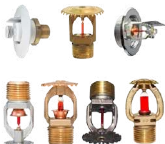
BOQUILLAS ROCIADORAS
