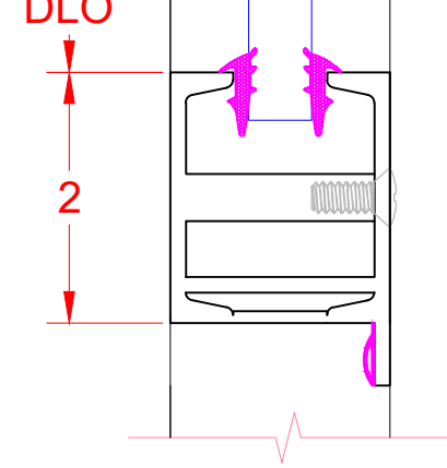
DOOR HEADER
