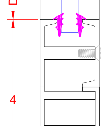
OPTIONAL SILL
