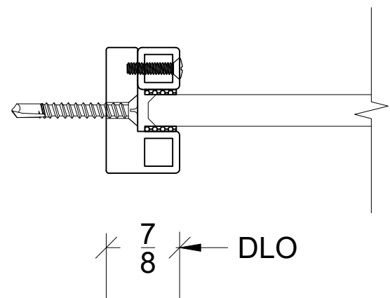
JAMB DETAIL
