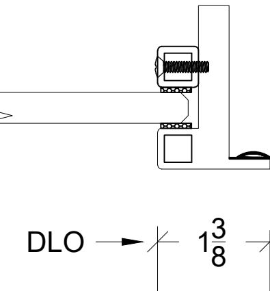
DOOR JAMB DETAIL
