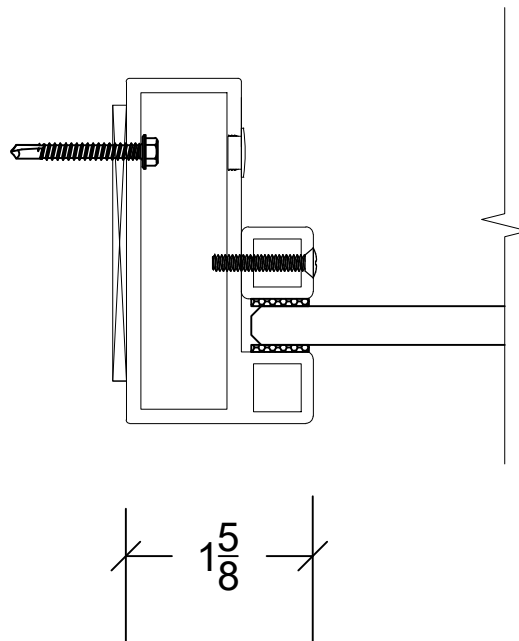
JAMB DETAIL
