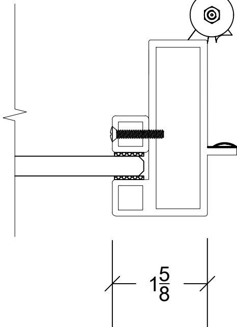
DOOR JAMB DETAIL
