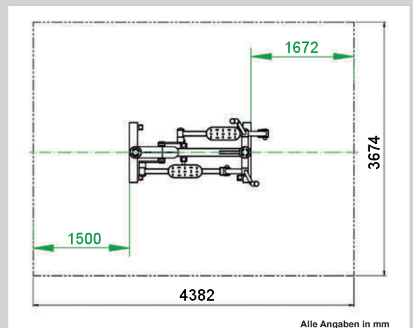
Draufsicht mit Bewegungsfläche
