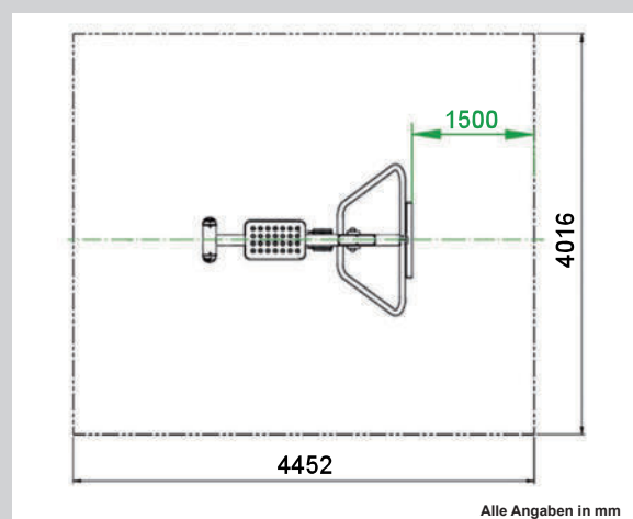
Draufsicht mit Bewegungsfläche
