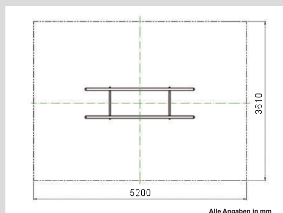
Draufsicht mit Bewegungsfläche
