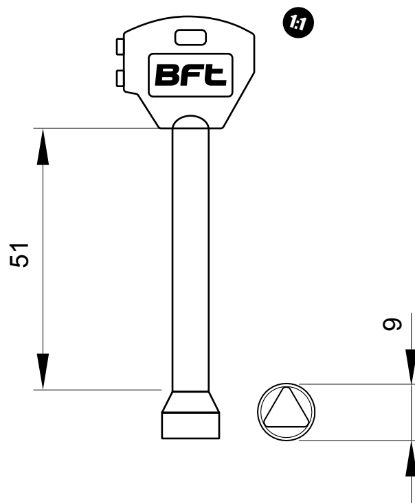
TRIANGOLARE IN METALLO MOD. LUNGO
