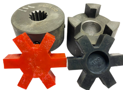
Acople L100 lado bomba, lado motor diesel y araña en cuacho o poliuretano
