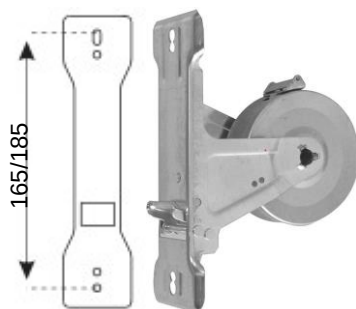
AVVOLGITORE INT. 165/185mm
