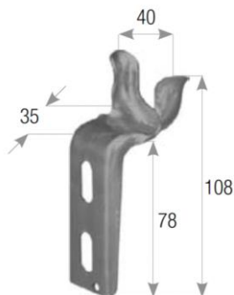
SUPPORTO A CASSONETTO DA 35mm
