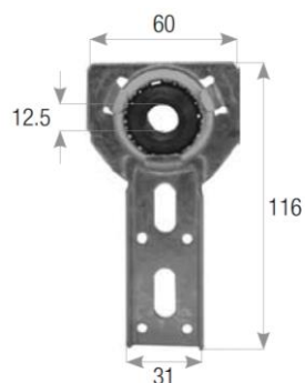
SUPPORTO A CASSONETTO DRITTO CON CUSCINETTO
