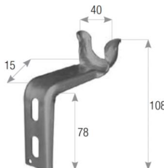
SUPPORTO A CASSONETTO DA 90mm
