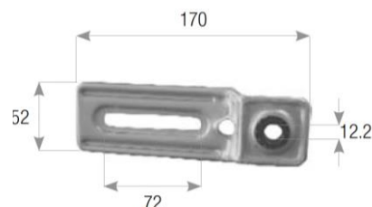
STAFFA ORIZZONTALE
