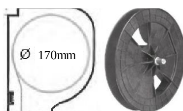
PULEGGIA PVC DIAM. 170mm
