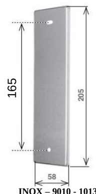
TAPPO LATERALE CASSONETTO A SCATTO
