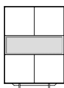
NYR VIT LAAG NR. 320 B 1128 mm / H 1570 mm / D 475 mm
