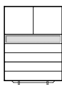
NYR VIT LAAG NR. 314 B 1128 mm / H 1570 mm / D 475 mm
