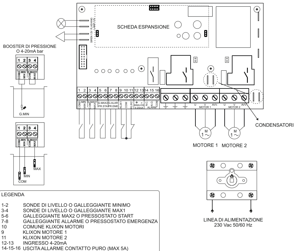
COLLEGAMENTO TRASDUTTORE DI PRESSIONE 4-20mA
