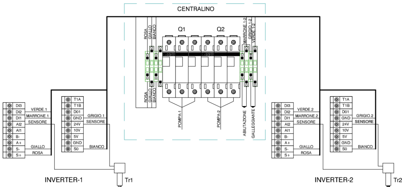
FIG.2: COLLEGAMENTI ELETTRICI PER GRUPPI CON INVERTER PDH TRIFASE – Gruppi GP-2E....
