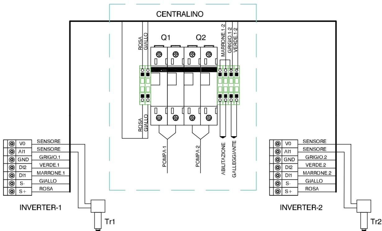
FIG.2: COLLEGAMENTI ELETTRICI PER GRUPPI CON INVERTER PDH TRIFASE – Gruppi GP-2E....
