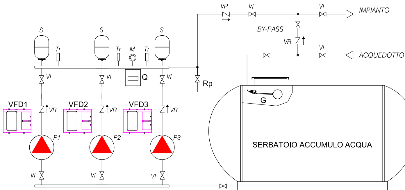
SCHEMA COLLEGAMENTI IDRAULICI PER INSTALLAZIONE SOTTO BATTENTE
