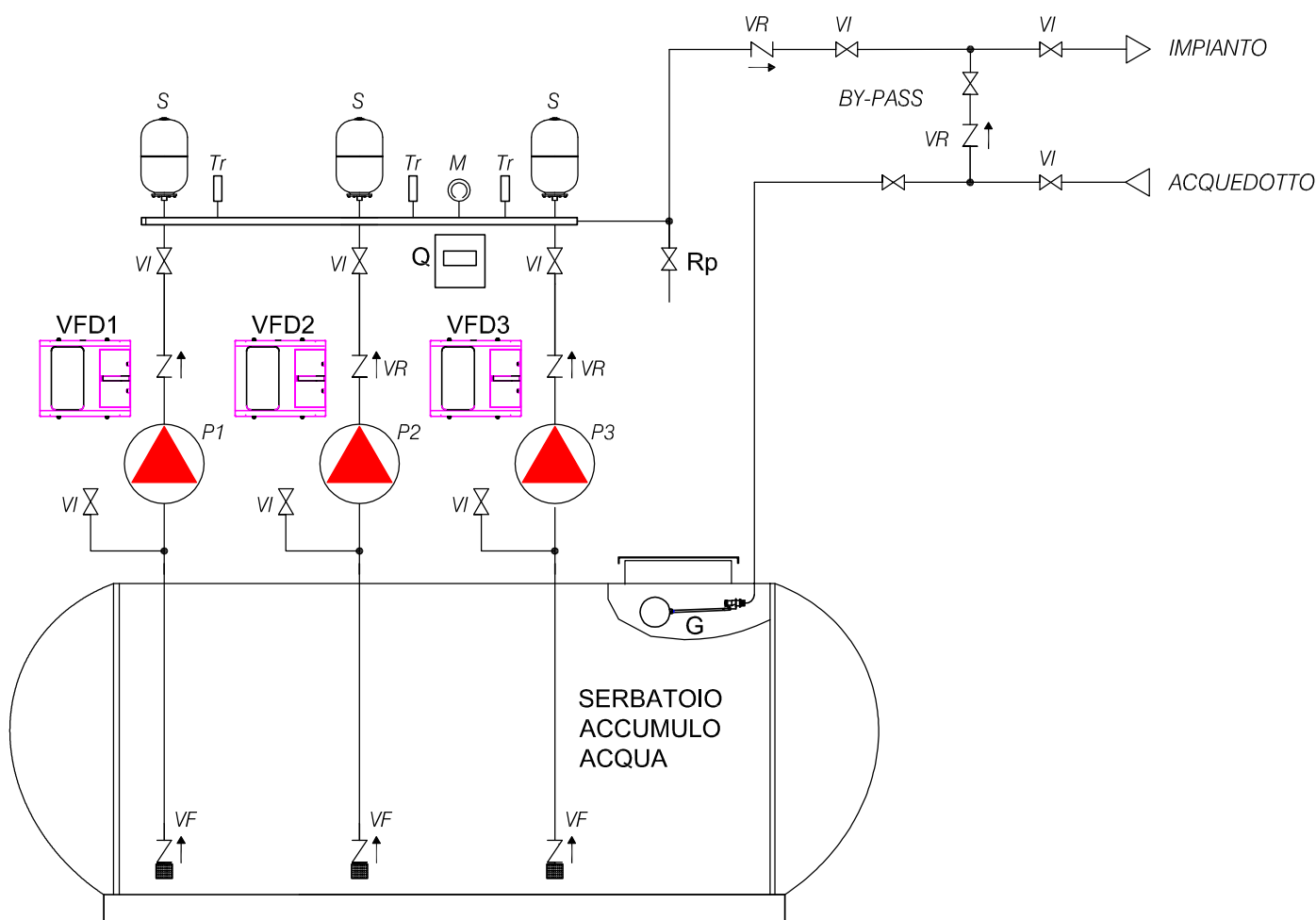
SCHEMA COLLEGAMENTI IDRAULICI PER ASPIRAZIONE POMPE NEGATIVA
