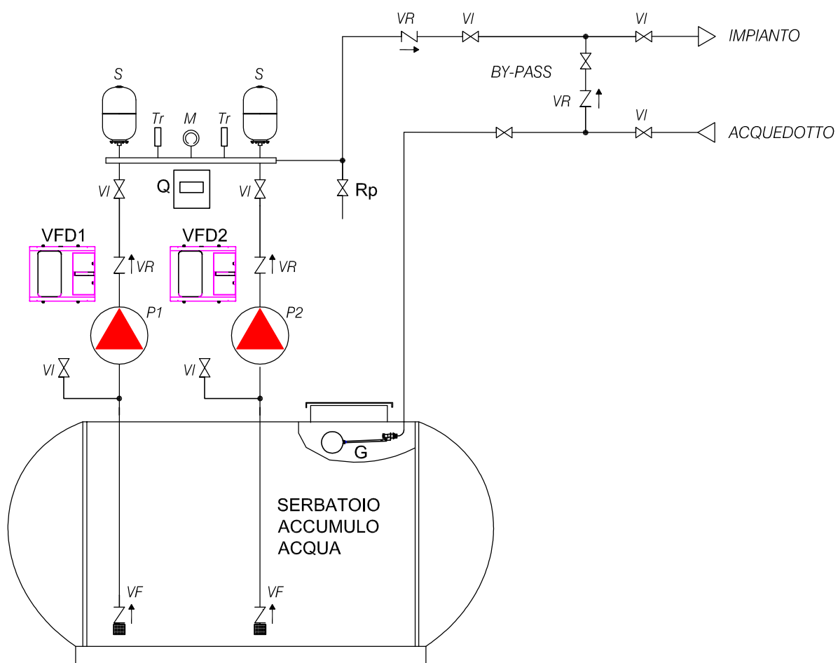
SCHEMA COLLEGAMENTI IDRAULICI PER ASPIRAZIONE POMPE NEGATIVA
