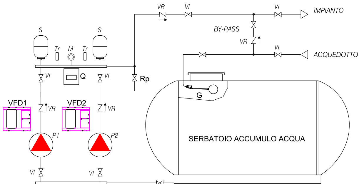
SCHEMA COLLEGAMENTI IDRAULICI PER INSTALLAZIONE SOTTO BATTENTE
