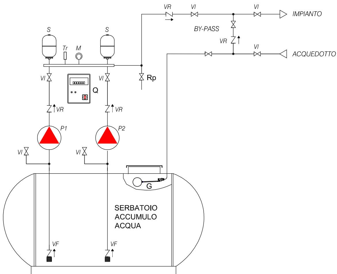
SCHEMA COLLEGAMENTI IDRAULICI PER ASPIRAZIONE POMPE NEGATIVA
