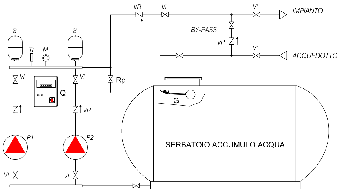
SCHEMA COLLEGAMENTI IDRAULICI PER INSTALLAZIONE SOTTO BATTENTE
