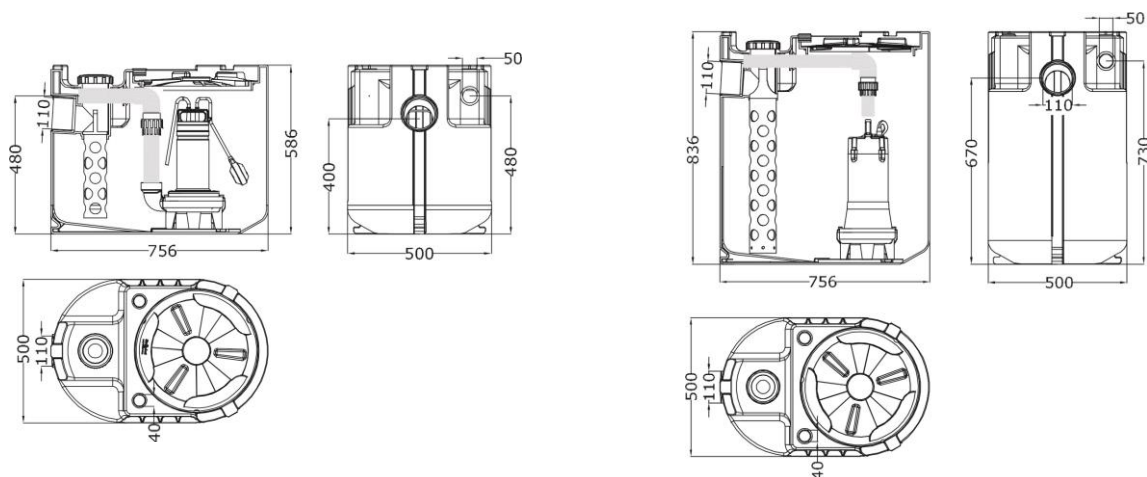
Stazione di sollevamento LEO-LIFT 100X
