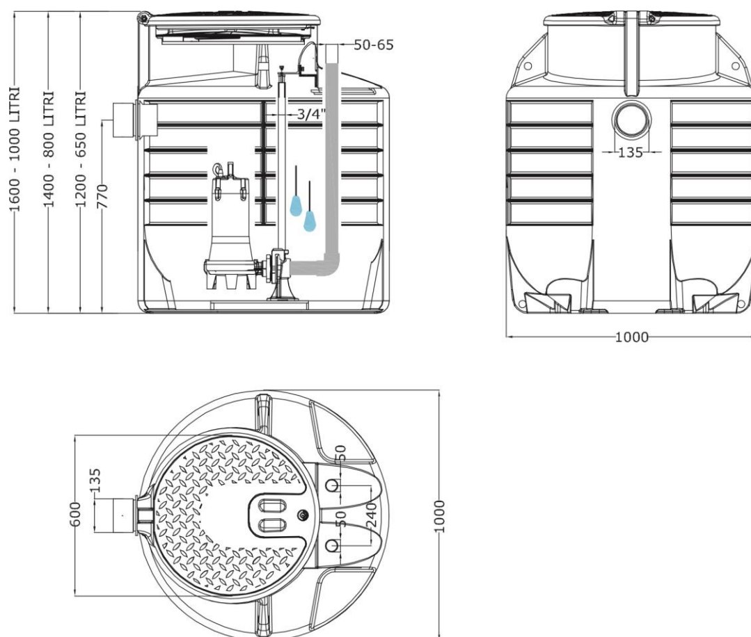
Stazione di sollevamento LEO-LIFT650X con pompa 50SWP 12-15
