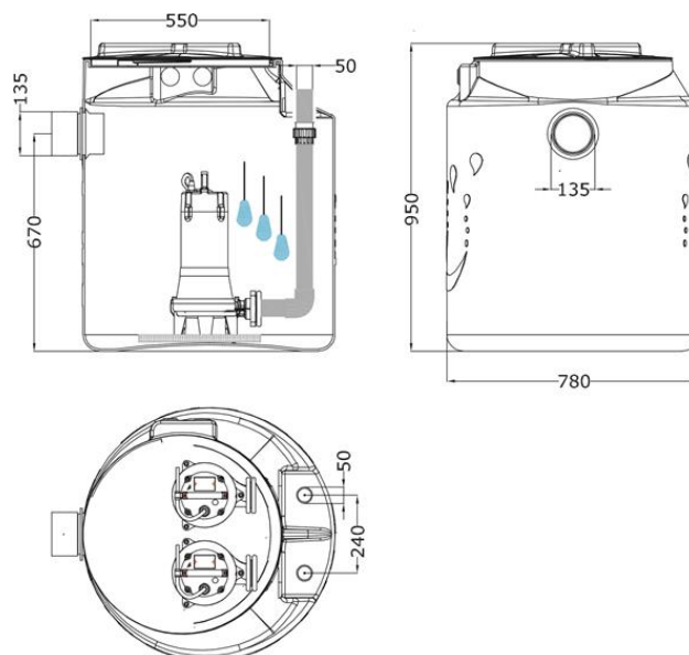
Stazione di sollevamento LEO-LIFT 400X
