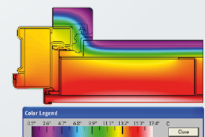
VERSIONE TERMO-ACUSTICA
