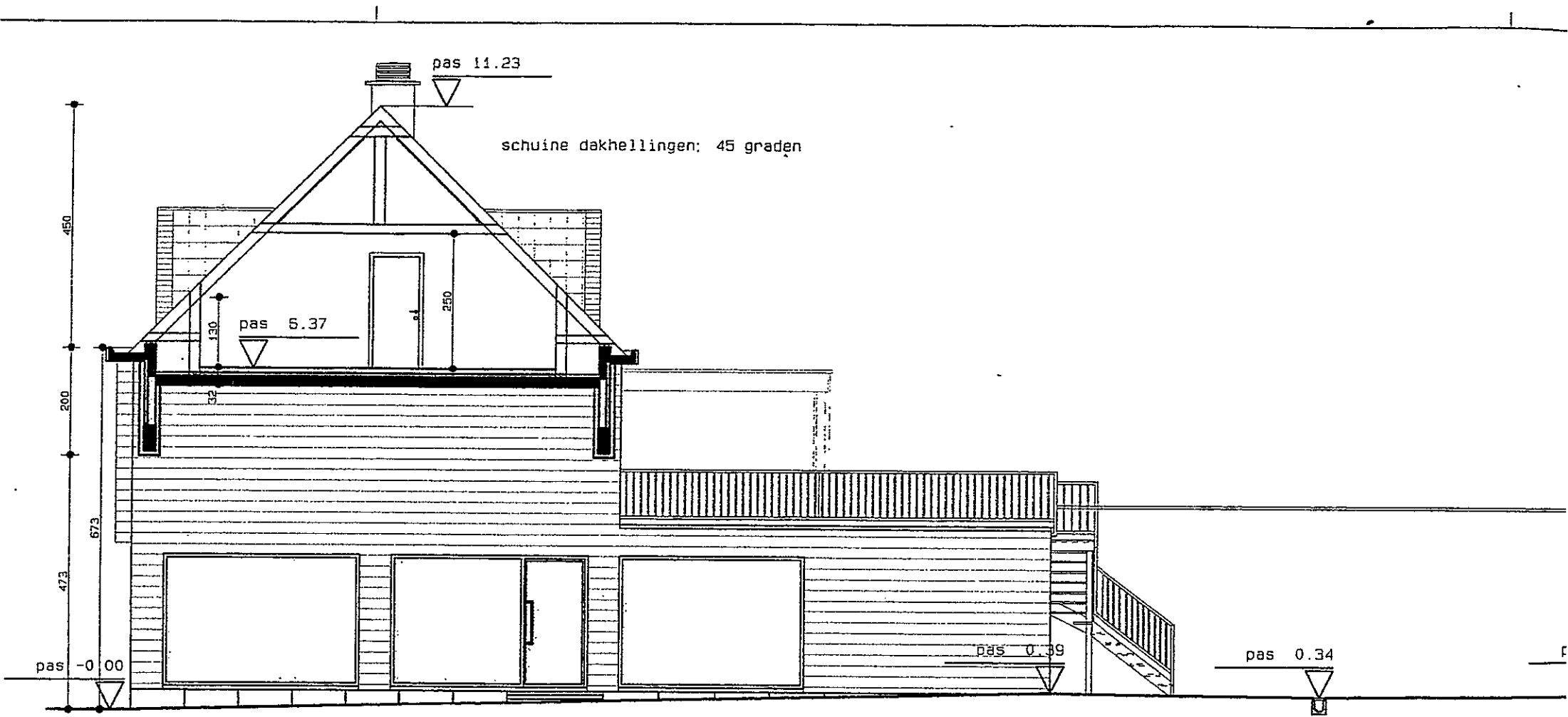
SNEDE A - B en ZIJGEVEL RECHTS
