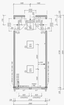
1023211 Skrifstofueining Stök eining
