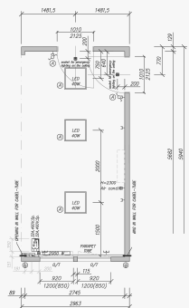
1023214 Endaeining Hægri endi
