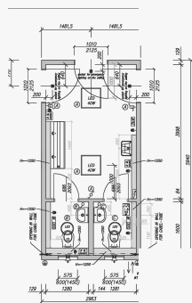
1024215 Snyrtieining Salerni og þvottaaðstaða
