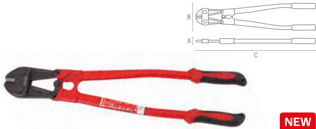
► CORTA-VARÕES 6009N
