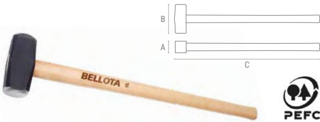
▶ MAÇA 5200
