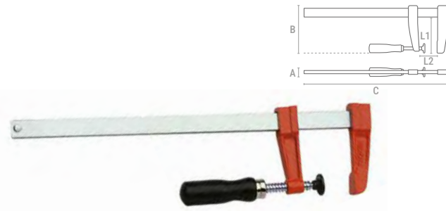
▶ SARGENTO EBANISTERIA 51200
