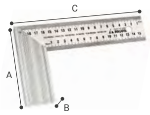
► ESQUADRO INOXIDÁVEL 50215
