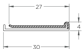
RT-052 (Portaprecio plano 55 mm Cristal)
