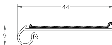
RT-029 (Portaprecio Blister 40 mm)
