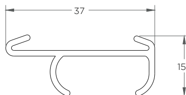
RT-084 (Base Oxxo para enganche central)
