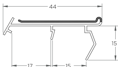
RT-043 (Portaprecio enganche invertido 40 mm)
