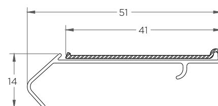
RT-062 (Portaprecio IMG)
