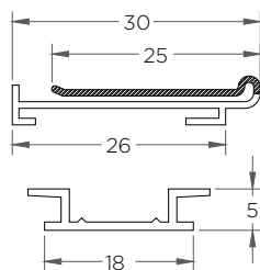
RT-056 (Portaprecio Universal 30 mm )
