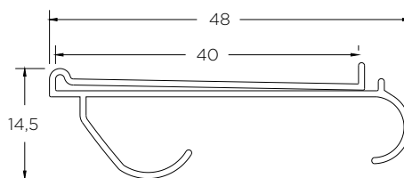
RT-118 (Portaprecio Enganche en C)
