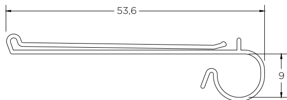
RT-125 (Portaprecio Blister 40x9 mm)
