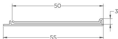
RT-052 (Portaprecio plano 55 mm Cristal)
