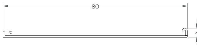
RT-045 (Portaprecio plano 80 mm Cristal)
