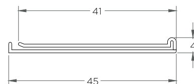
RT-045 (Portaprecio plano 80 mm Cristal)
