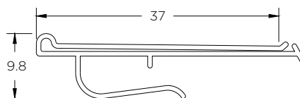
RT-061 (Portaprecio enganche inferior)
