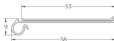
RT-035 (Portaprecio Blister 55 mm Cristal)
