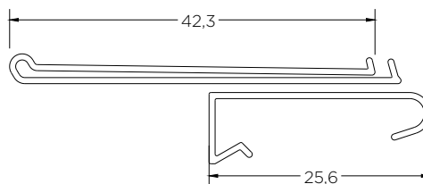
RT-121 (Portaprecio Triextruido riel C)
