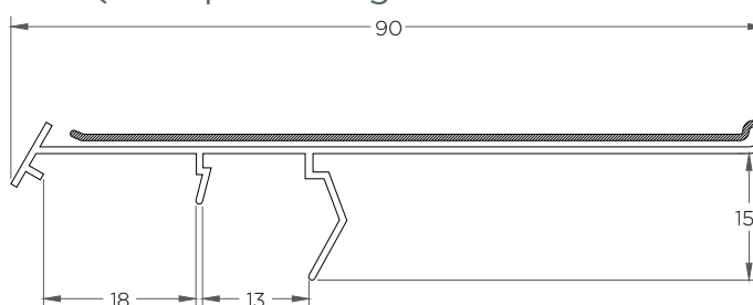
RT-044 (Portaprecio enganche invertido 80mm)
