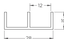
RT-048 (Carrilera 28 mm)
