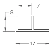
PT-011 (F 17 mm PS)
