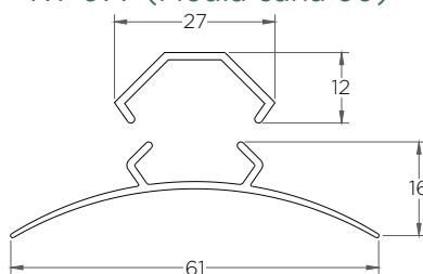
RT-077 (Media caña 60)
