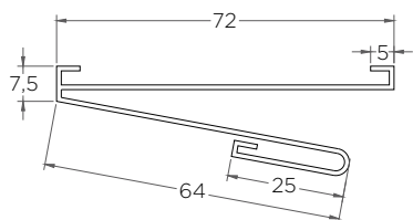
ET-022 (Z Doria poliestireno)
