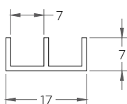
PT-009 (Carrilera 17 mm PS)
