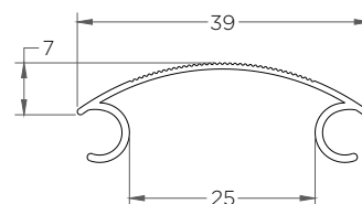
ET-020 (Enganche Legajador)
