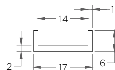
BT-008 (Cinta borde plano 14 mm)
