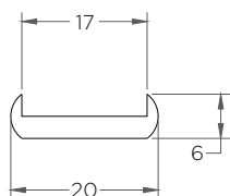
ET-028 (Cinta borde curvo 17 mm)
