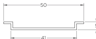
RT-057 (Patín 50 mm)
