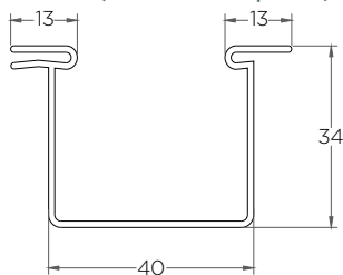
ET-016 (Porta lámpara)
