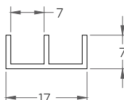
RT-022 (Carrilera 17 mm)
