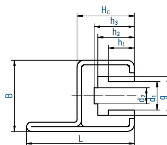
Type CKG 14H
