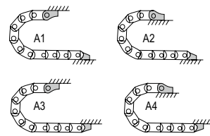
接头安装方式 Connector mounting way
