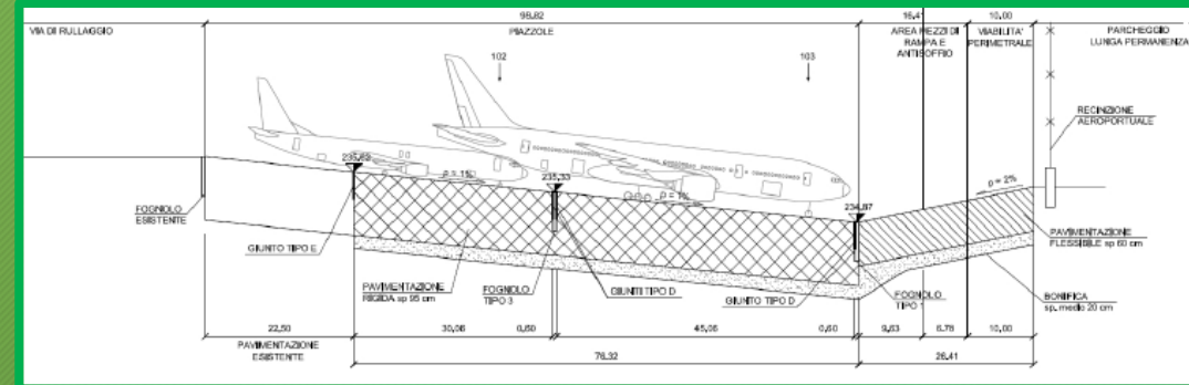
Sezione trasversale pista
