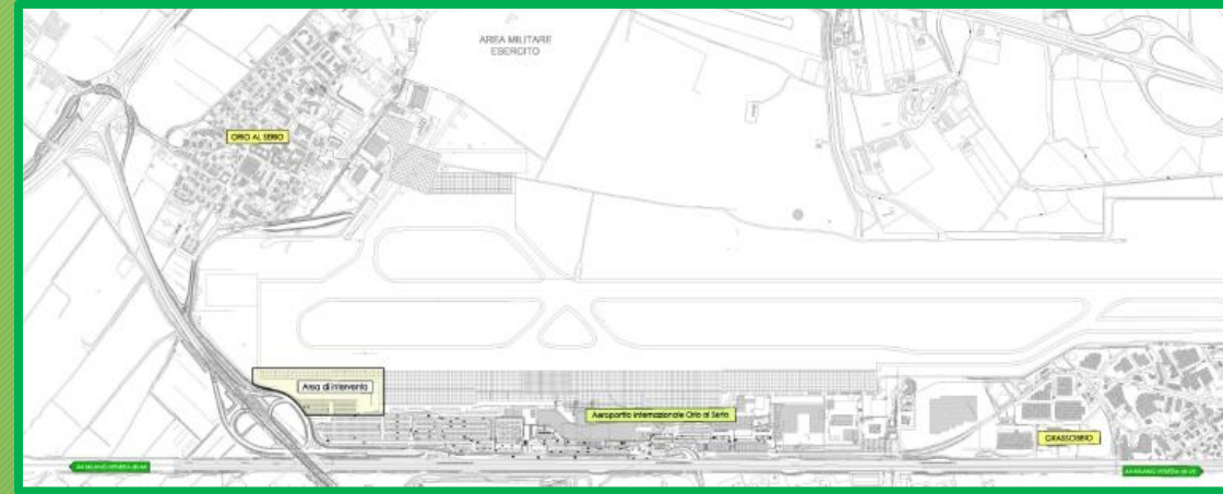
Planimetria segnaletica
