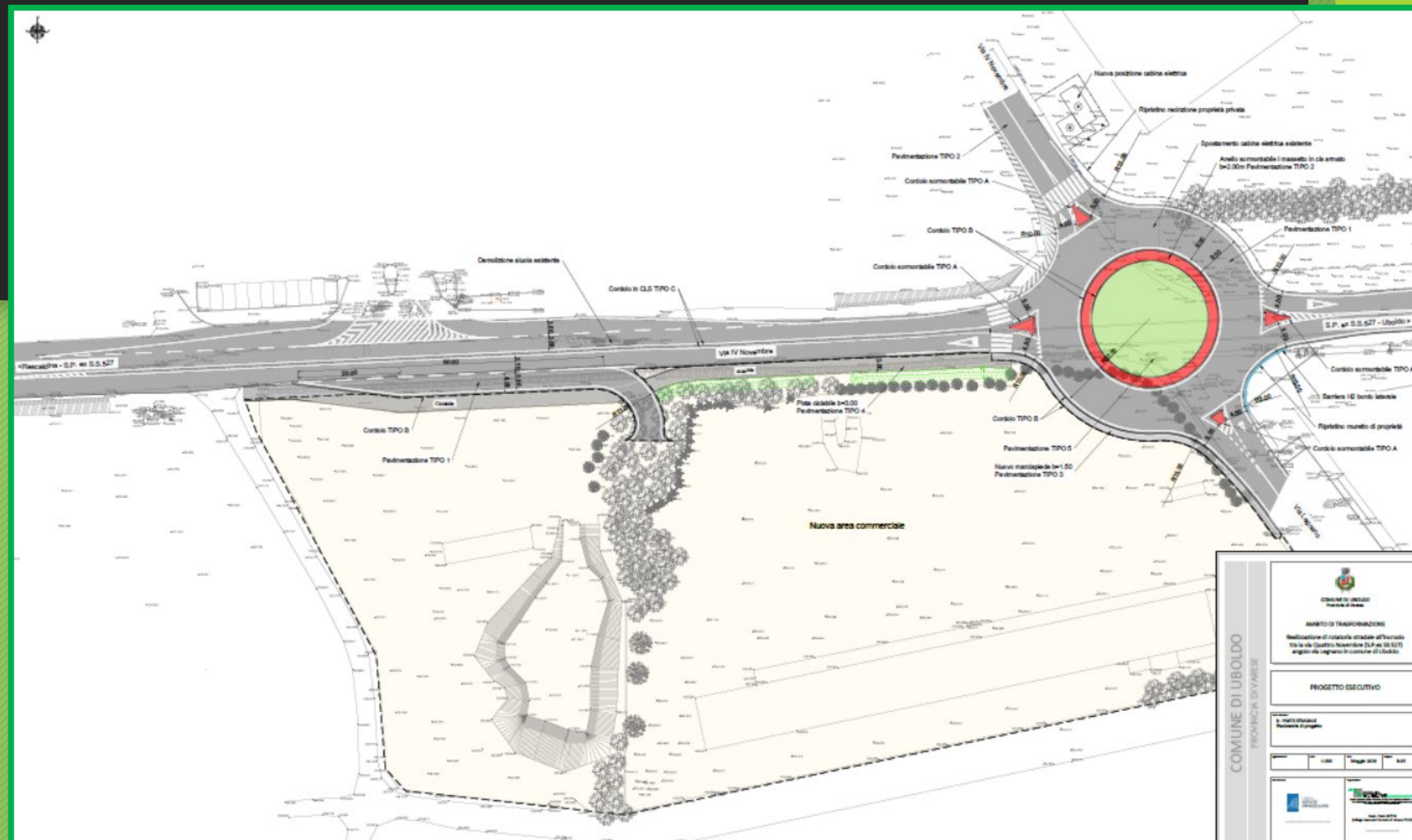
Planimetria di progetto
