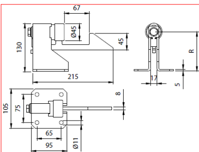
ARRESTO DI FINE CORSA REGOLABILE A FISSARE ZINCATO
