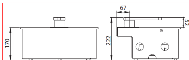
GRUPPO CASSA DI FONDAZIONE CATAFORESI compresa di kit bracci e leverismi
