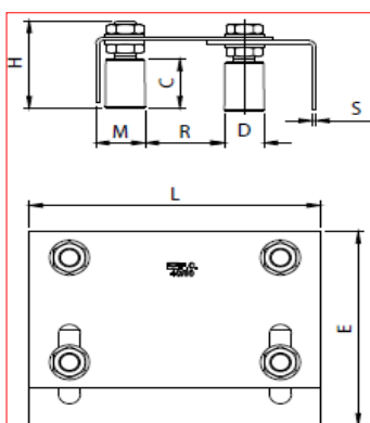
PIASTRA GUIDA CANCELLO A DOPPIA REGOLAZIONE ZINCATA
