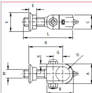
CARDINE A FASCETTA CON INGRASSATORE E DADO REG. ZINCATO
