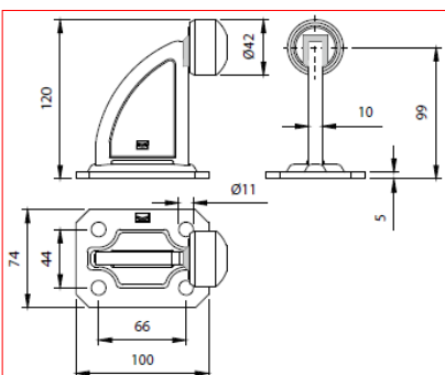
ARRESTO DI FINE CORSA CON BASE A FISSARE ZINCATO
