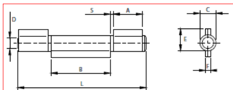
CERNIERA A 3 ALI PERNO SFILABILE
