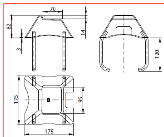
BATTENTE D'ARRESTO A CEMENTARE CON ANCORANTI
