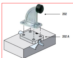
BATTENTE D'ARRESTO A FISSARE ZINCATO
