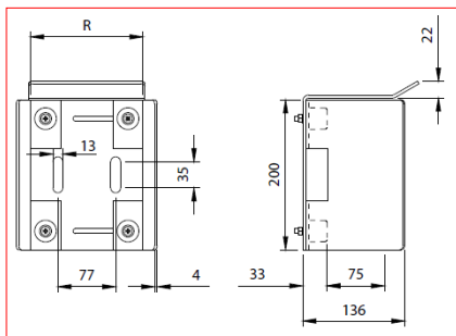
INCONTRO APERTO REGOLABILE CON TAPPI AMMORTIZZATORI ZINCATO
