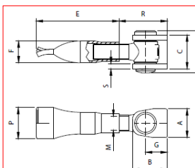
CARDINE CON ALI A CEMENTARE ZINCATO
