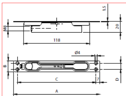
CATENACCIO AD INCASSO A UNA MANDATA ZINCATO CON LEVA ZINCATA
