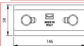
MINIPIASTRA GUIDA CANCELLO ZINCATO
