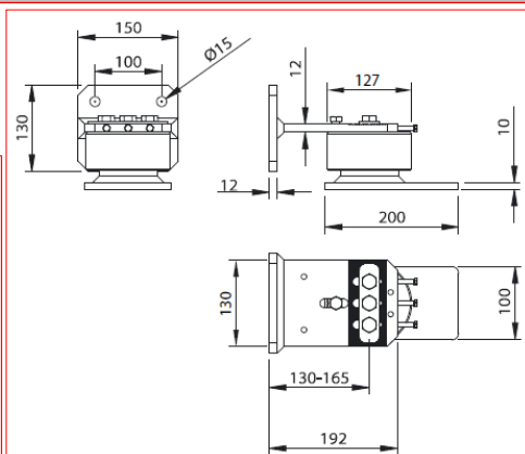
CARDINE SUPERIORE PESANTE DOPPIA REGOLAZIONE E PIASTRA A FISSARE ZINCATO
