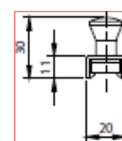
INCONTRO PER CATENACCIO (art. 740) ZINCATO
