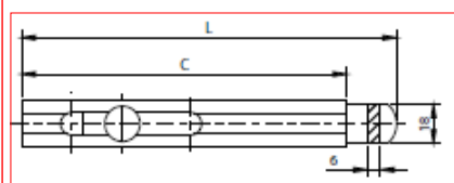
CATENACCIO MEDIO A SALDARE ZINCATO
