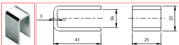
INCONTRO PER CATENACCIO (art. 740) ZINCATO
