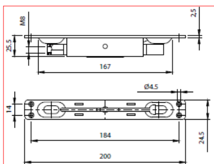
CATENACCIO AD INCASSO DOPPIA MANDATA ZINCATO CON LEVA IN OTTONE
