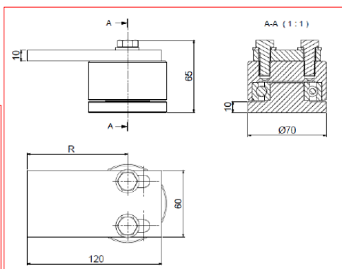
CARDINE SUPERIORE CON PIASTRA ACCIAIO INOX
