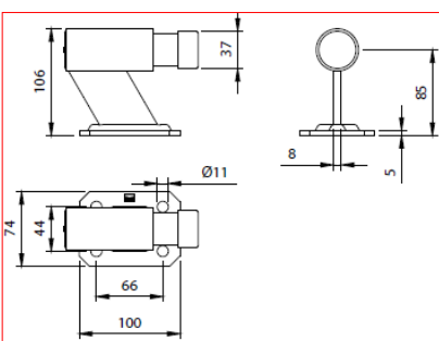
ARRESTO DI FINE CORSA AMMORTIZZATO CON BASE A FISSARE ZINCATO
