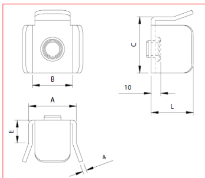
INCONTRO SUPERIORE CON TAPPO AMMORTIZZATORE ZINCATO
