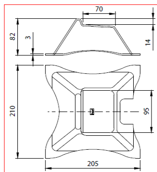
BATTENTE D'ARRESTO A FISSARE ZINCATO
