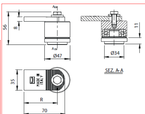
CARDINE SUPERIORE CON CUSCINETTO E PIASTRA ZINCATO
