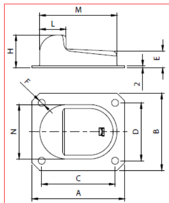
BATTENTE D'ARRESTO A CEMENTARE ZINCATO
