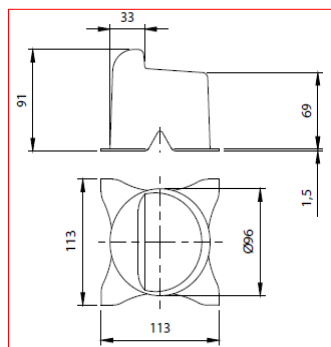
BATTENTE D'ARRESTO A CEMENTARE CON ANCORANTI
