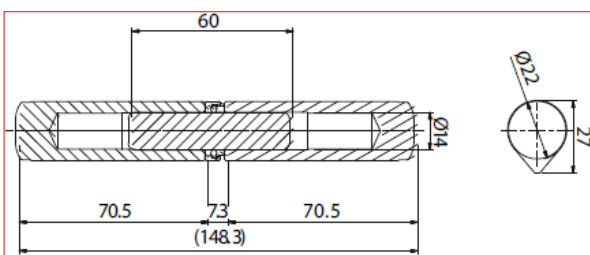
CERNIERA FUTURA NON ZINCATA CON PERNO IN OTTONE SFILABILE CON CUSCINETTO
