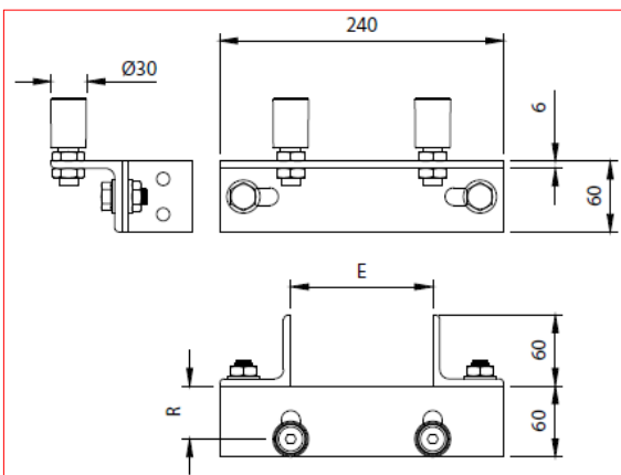
PIASTRA GUIDA CANCELLO INTERNA REGOLABILE A FISSARE ZINCATA
