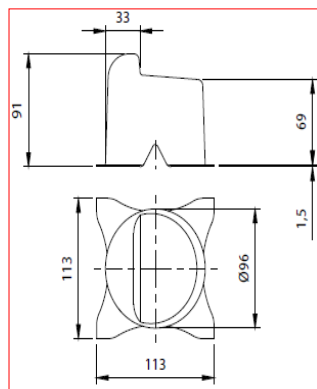
BATTENTE D'ARRESTO A CEMENTARE ZINCATO
