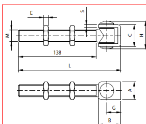
CARDINE CON ALI E BUSSOLA ZINCATO
