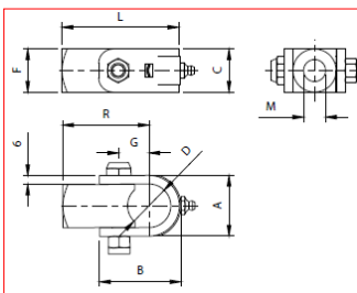
CORPO CARDINE A FASCETTA CON INGRASSATORE PER BARRE FILETTATE ZINCATO
