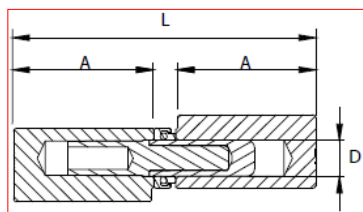
CERNIERA FUTURA NON ZINCATA CON PERNO RINFORZATO RIVESTITO IN OTTONE CON CUSCINETTO
