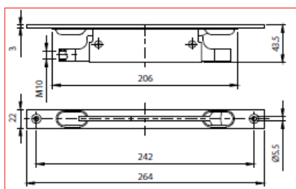
CATENACCIO AD INCASSO PER PORTE BLINDATE DOPPIA MANDATA ZINCATO CON LEVA IN OTTONE NICHELATA
