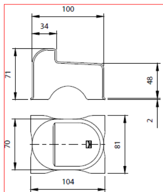
BATTENTE D'ARRESTO A CEMENTARE INOX
