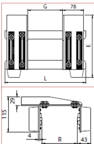
PIASTRA GUIDA CANCELLO REGOLABILE GIGANTE ZINCATA
