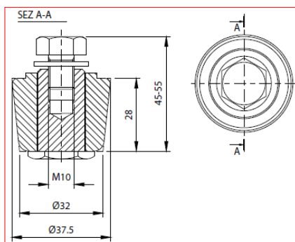
OLIVA CONICA IN NYLON BULLONE ZINCATO
