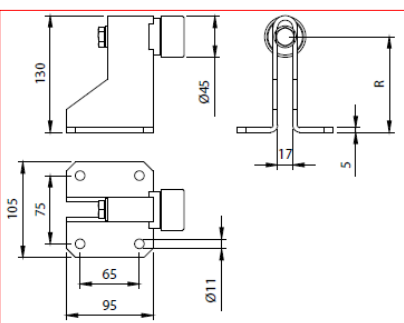
ARRESTO DI FINE CORSA REGOLABILE A FISSARE ZINCATO
