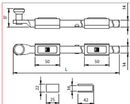
CATENACCIO PUNTA TONDA DA 14 ZINCATO
