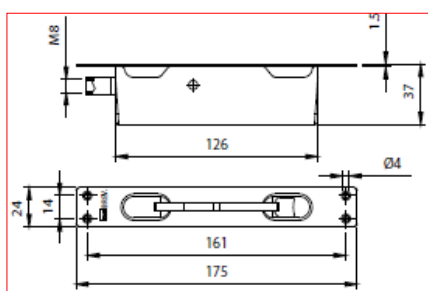
CATENACCIO AD INCASSO PER PORTE BLINDATE A UNA MANDATA ZINCATO CON LEVA IN OTTONE NICHELATA
