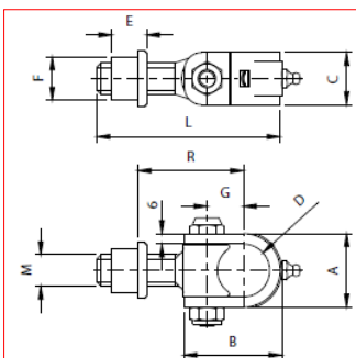
CARDINE A FASCETTA CON INGRASSATORE E BUSSOLA ZINCATO
