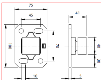
PIASTRA INFERIORE A FISSARE CON PERNO SFERICO ZINCATO
