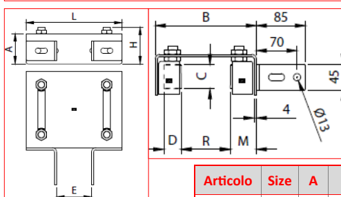
PIASTRA GUIDA CANCELLO REGOLABILE CON STAFFE ANGOLARI ZINCATA
