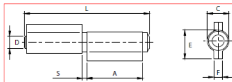
CERNIERA A 2 ALI PERNO SFILABILE
