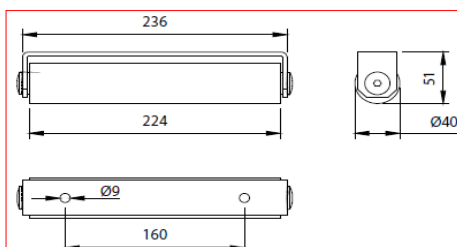
MAXI RULLO IN NYLON A FISSARE ZINCATO
