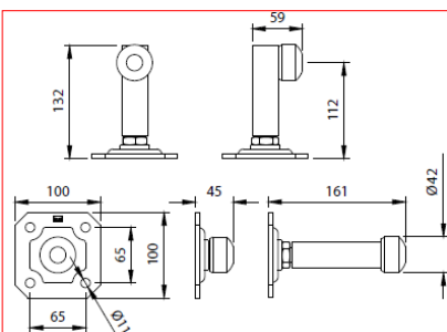
BATTENTE TRIS A FISSARE TRIPLA FUNZIONE ZINCATO
