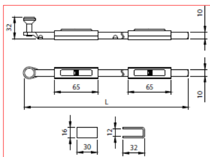
CATENACCIO PUNTA TONDA DA 10 ZINCATO
