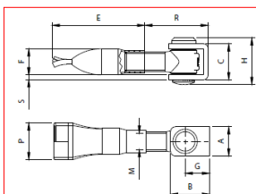
CARDINE CON CAVALLOTTO A CEMENTARE ZINCATO
