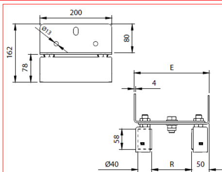
PIASTRA A DOPPIA REGOLAZIONE A FISSARE PER CANCELLI A DOPPIA COLONNA ZINCATA
