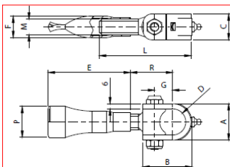
CARDINE A FASCETTA A CEMENTARE CON INGRASSATORE ZINCATO
