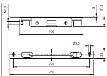
CATENACCIO AD INCASSO PER PORTE BLINDATE A DOPPIA MANDATA ZINCATO CON LEVA IN OTTONE NICHELATA
