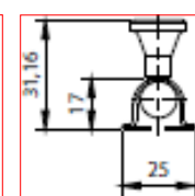
CATENACCIO A SALDARE ASTA TONDA 12 mm ZINCATO
