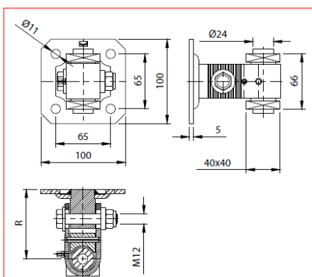
CARDINE "GIULIANO" ZINCATO
