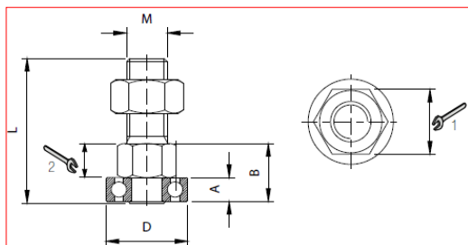
PERNO CON CUSCINETTO BULLONE ZINCATO
