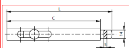
CATENACCIO LEGGERO 14 mm ZINCATO
