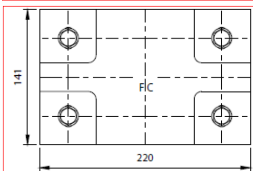
PIASTRA GUIDA CANCELLO REGOLAB. ZINCATO
