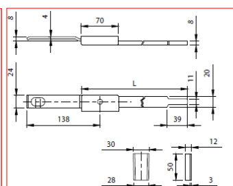
CATENACCIO MEDIO A SALDARE ZINCATO
