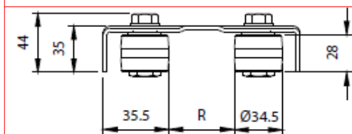
PIASTRA GUIDA CANCELLO REGOLAB. INOX
