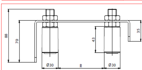
MINIPIASTRA GUIDA CANCELLO ZINCATO
