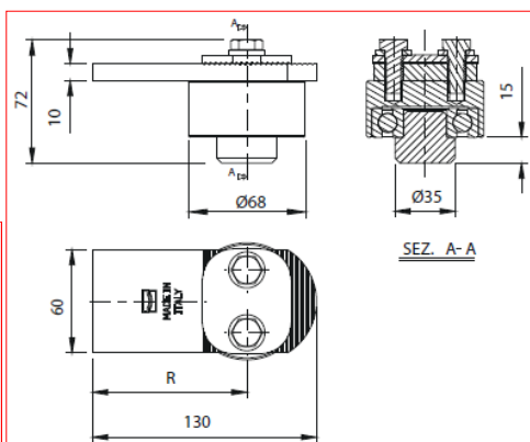
CARDINE SUPERIORE CON PIASTRA A FISSARE ZINCATO
