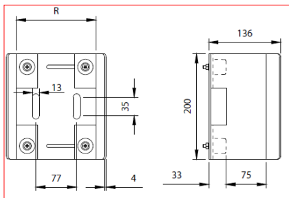
INCONTRO CHIUSO REGOLABILE CON TAPPI AMMORTIZZATORI ZINCATO
