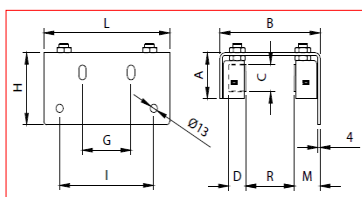
PIASTRA GUIDA CANCELLO REGOLABILE CON ALA LUNGA A FISSARE ZINCATA
