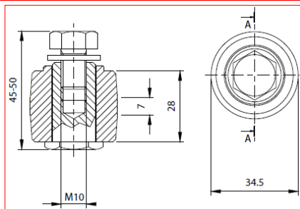
OLIVA IN NYLON BULLONE ZINCATO
