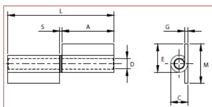
CERNIERA 2 ALI PIANE CON PERNO SFILABILE
