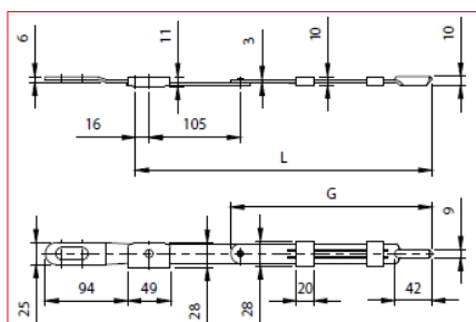
CATENACCIO A LEVA A PUNTA ARROTONDATA ZINCATO
