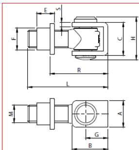
CARDINE CON CAVALLOTTO E BUSSOLA ACCIAIO INOX
