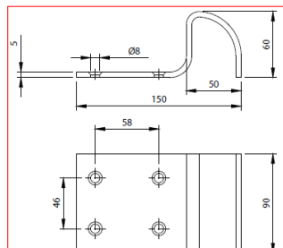
BATTENTE D'ARRESTO A FISSARE ZINCATO
