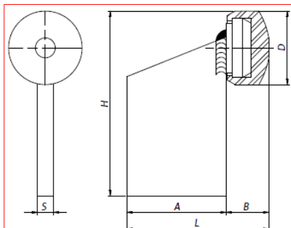
ARRESTO DI FINE CORSA INOX
