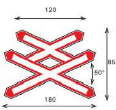
FIG. 10/b ART. 87 DOPPIA CROCE DI S. ANDREA obbligatorio in pellicola classe II
