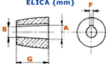
DIMENSIONI MOZZO ELICA (mm)
