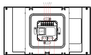
④ 後視圖
