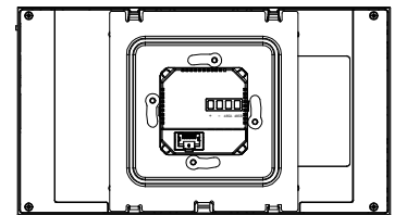
④ 後視圖
