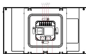
④ 後視圖
