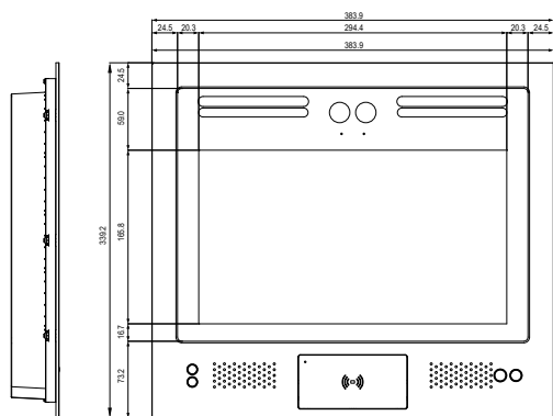
① 正視圖
