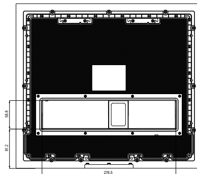
④ 後視圖
