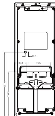
④ 後視圖
