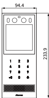
① 正視圖
