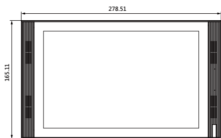
① 正視圖
