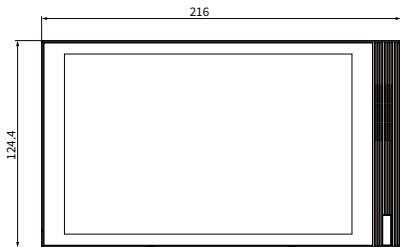
① 正視圖
