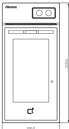
① 正視圖
