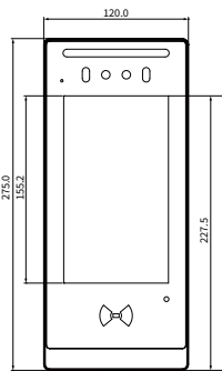
① 正視圖
