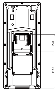
④ 後視圖
