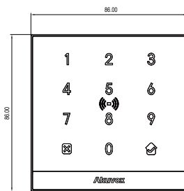
① 正視圖
