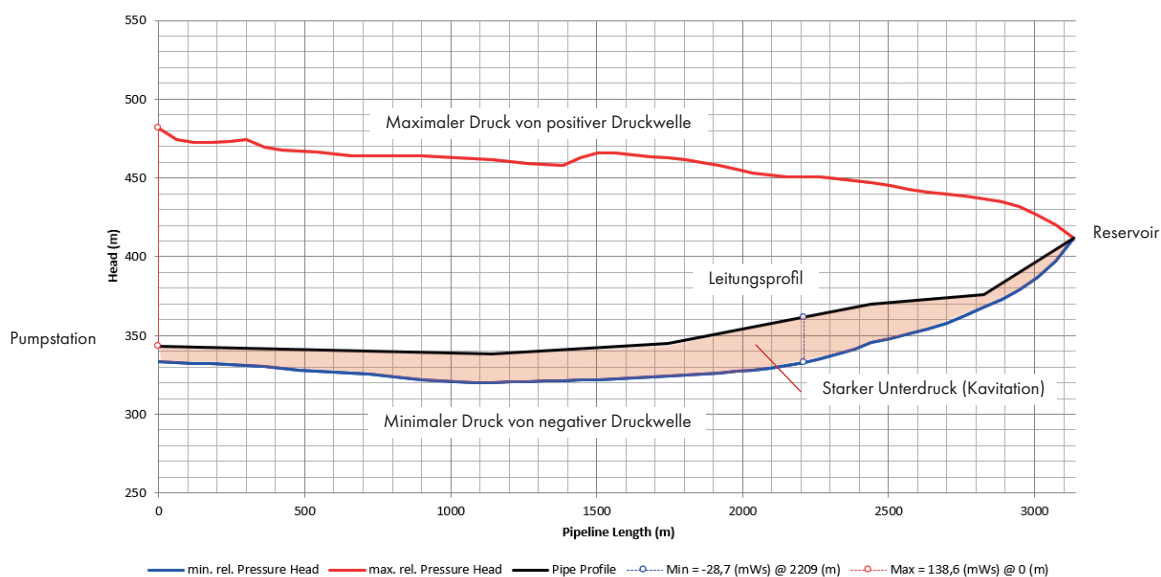
Druckverlauf über das ganze Längen-/Höhenprofil ohne Sicherheitselement
