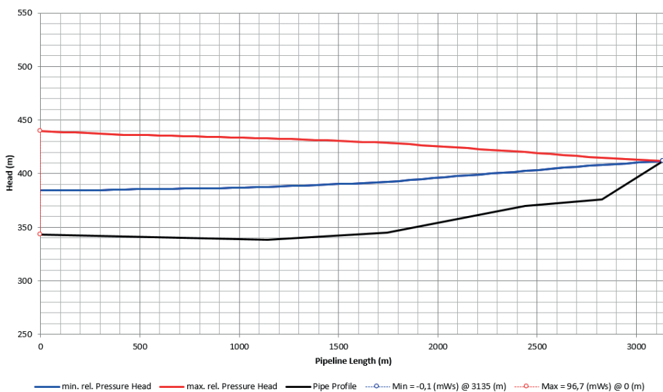
Druckverlauf über das gesamte Längen-/Höhenprofil mit Sicherheitselementen (Dämpfer)
