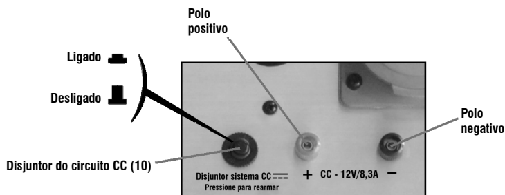
Fig. 17 – Disjuntor do circuito CC
