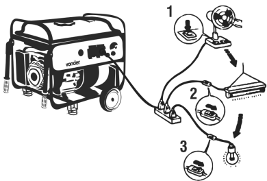
Fig. 4 – Secuencia de accionamiento de los equipamientos Normalmente, cargas inductivas y capacitivas, especialmente las motorizadas, tiene un grande pico de energía en el momento que son encendidas. La tabla 2 tiene como referencia algunos equipamientos que pueden ser conectados a los generadores
