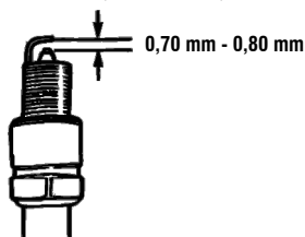
Fig. 27 – Folga a vela
