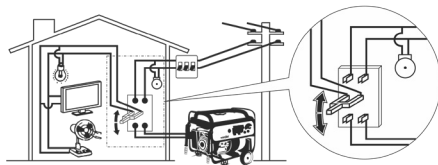
Fig. 2 – Ejemplo de conexión correcta
