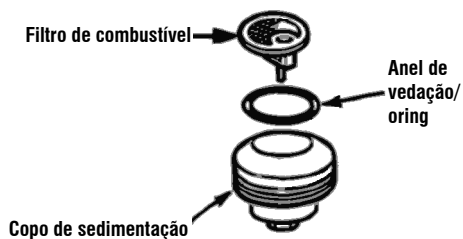
Fig. 25 – Limpeza dos componentes
