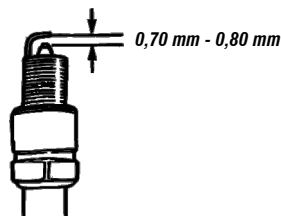
Fig. 27 – Distancia de la bujía
