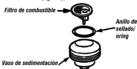
Fig. 25 – Limpieza de los componentes
