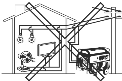
Fig. 3 – Ejemplo de conexión que nunca debe realizarse
