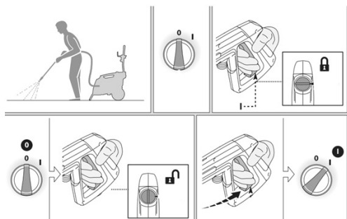
Fig. 7 – Uso da pistola
