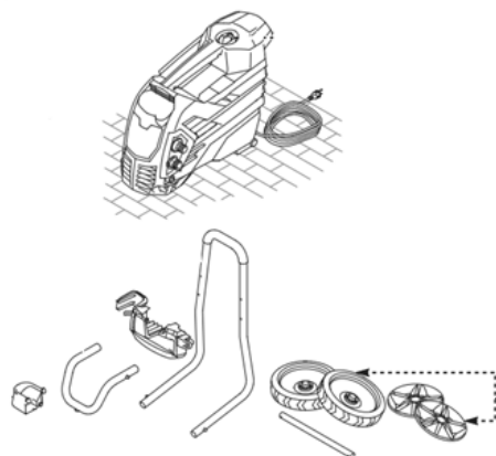
Fig. 2 – Montaje de los accesorios de la lavadora
