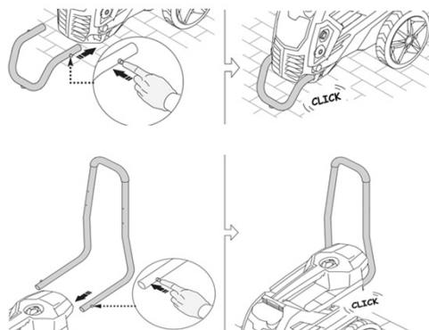
Fig. 4 – Instalando os suportes de transporte
