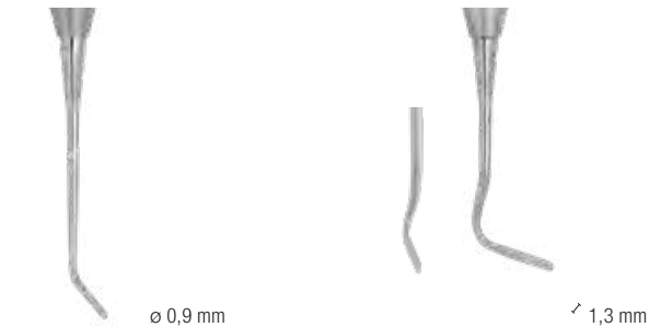
492/11 Goldstein N.11 Mini spatula / Plugger Mini spatola / Otturatore 492/14 Goldstein N.14 Mini spatula / Spatula Mini spatola / Spatola
