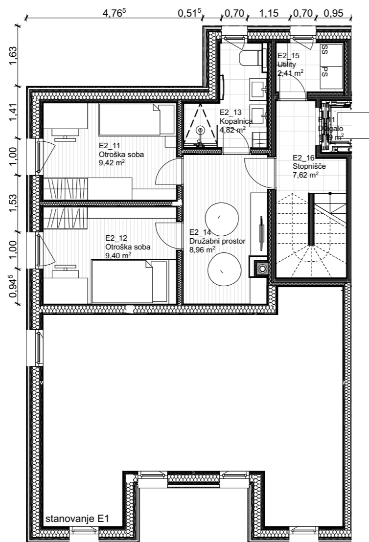
NADSTROPJE
