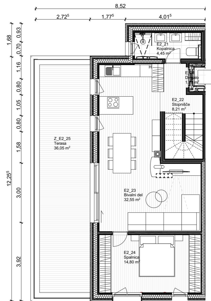
TERASNA ETAŽA
