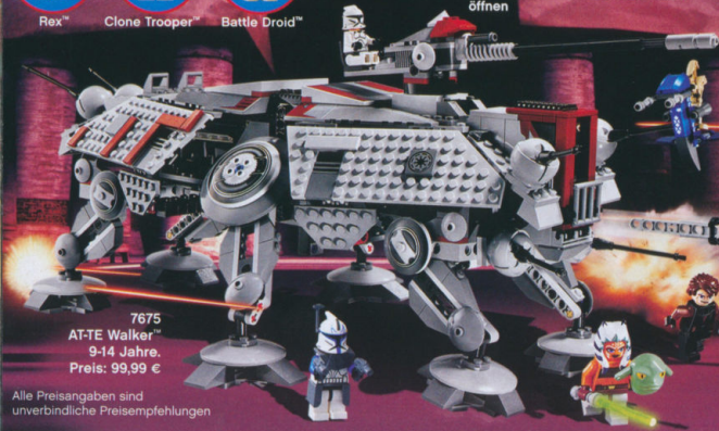
Schussfunktion
