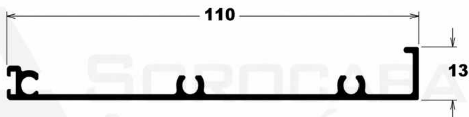
MN-002 0,669 Kg/m
