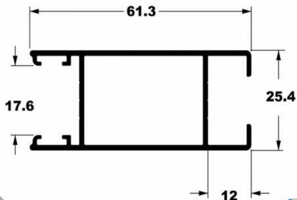
SU-238 0,714 Kg/m
