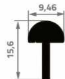
PR-003 0,166 Kg/m
