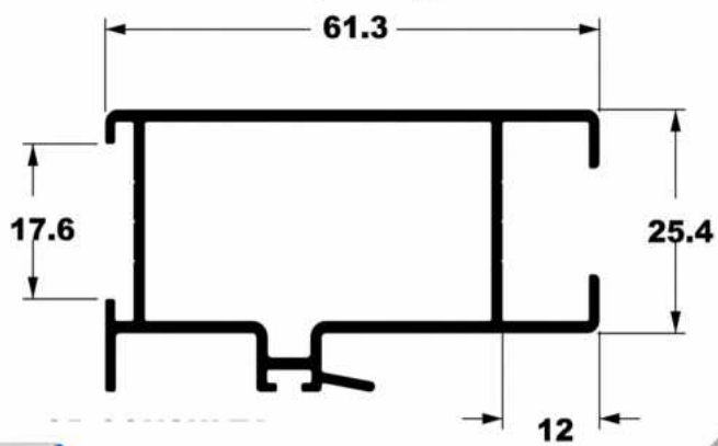
SU-239 0,783 Kg/m
