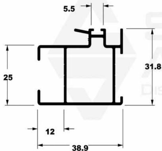
SU-238 0,714 Kg/m
