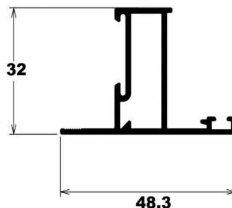
LG-085 0,529 Kg/m
