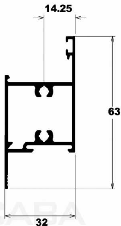
LG-076 0,765 Kg/m
