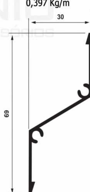
VZ-060 0,397 Kg/m
