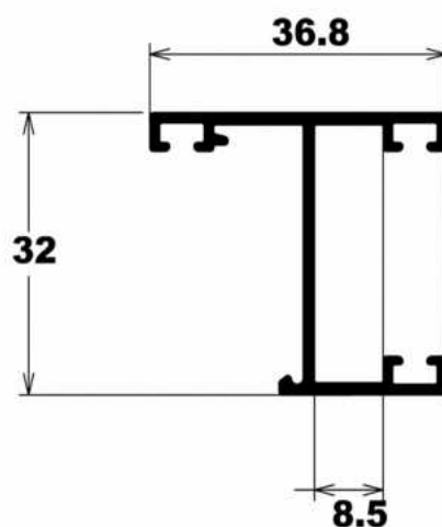
LG-068 0,405 Kg/m
