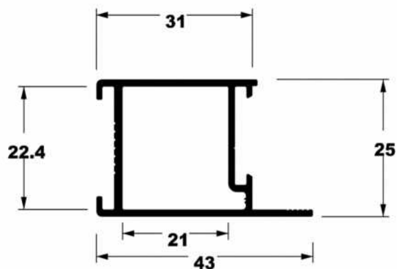
SU-292 0,640 Kg/m
