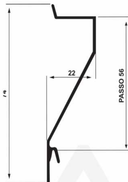
Z-203 0,301 Kg/m
