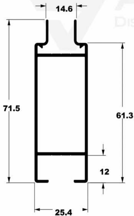
SU-240 0,771 Kg/m
