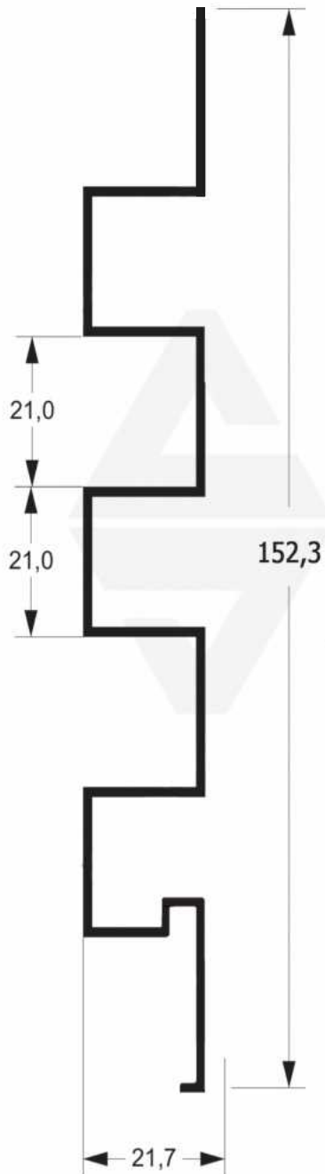
DP-074A 0,986 Kg/m
