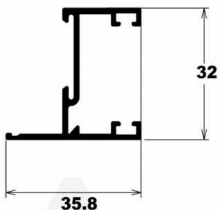
LG-083 0,449 Kg/m
