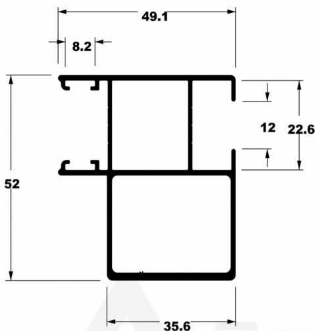
SU-060 0,978 Kg/m
