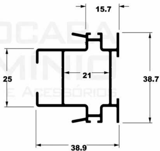
SU-239 0,783 Kg/m
