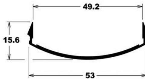
CG-074 0,270 Kg/m
