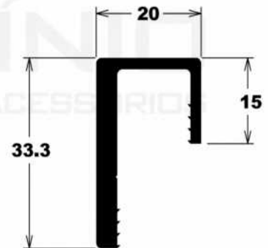
CG-075 0,520 Kg/m
