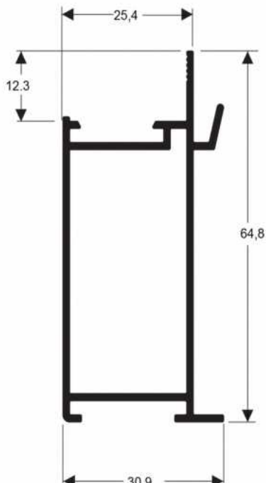
SU-243 0,713 Kg/m
