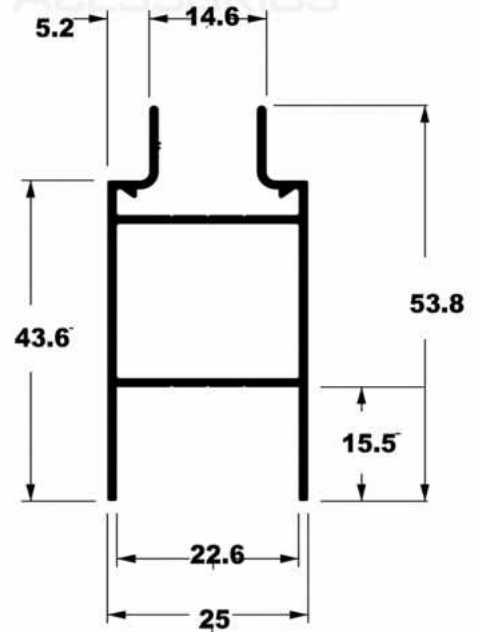
SU-191 0,533 Kg/m
