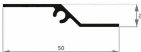
DV-113 0,253 Kg/m
