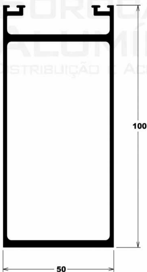
A-096 1,860 Kg/m
