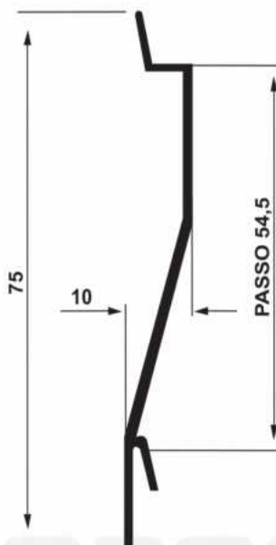
Z-201 0,271 Kg/m
