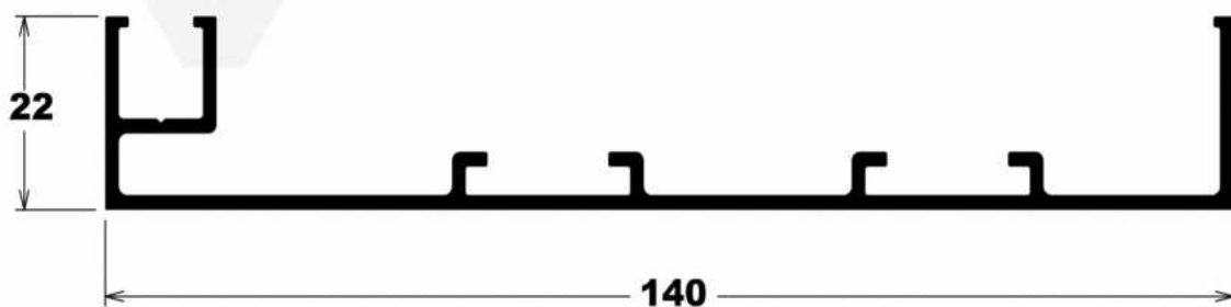
MN-003 1,093 Kg/m
