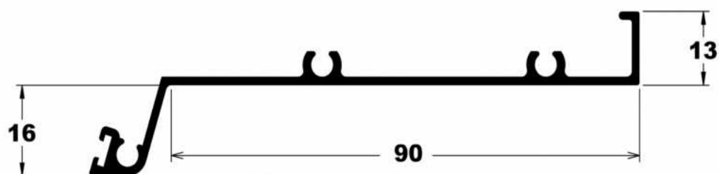
MN-023 0,688 Kg/m
