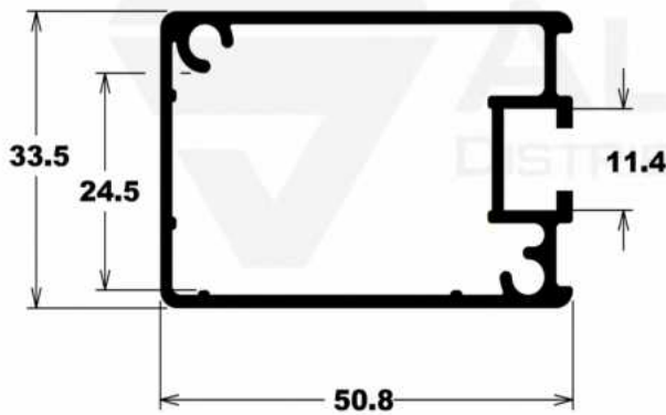
CG-077 0,842 Kg/m
