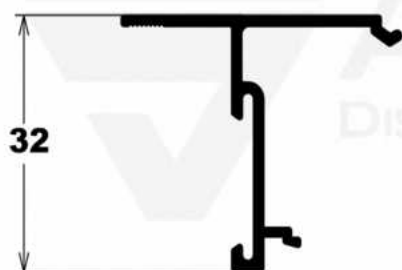
LG-077 0,835 Kg/m
