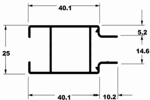
SU-190 0,543 Kg/m
