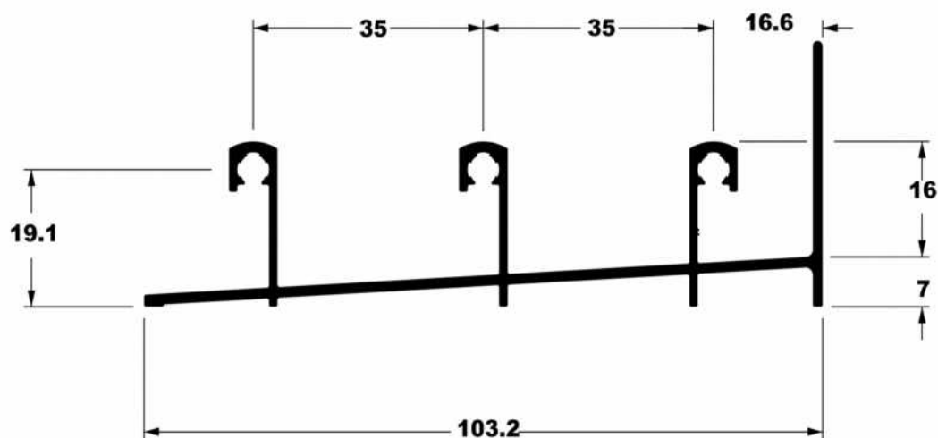
SU-230 0,954 Kg/m
