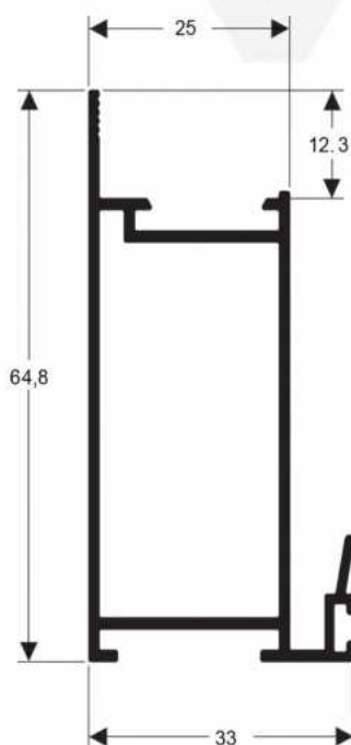
SU-242 0,742 Kg/m
