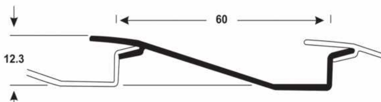
VZ-051 0,268 Kg/m
