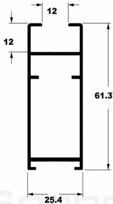
SU-241 0,734 Kg/m
