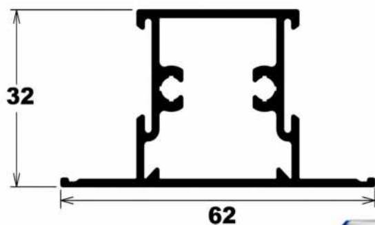
LG-079 0,770 Kg/m
