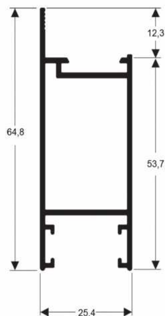
SU-245 0,672 Kg/m
