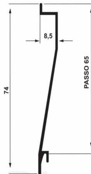
VZ-060 0,397 Kg/m
