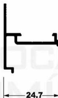
SU-292 0,640 Kg/m
