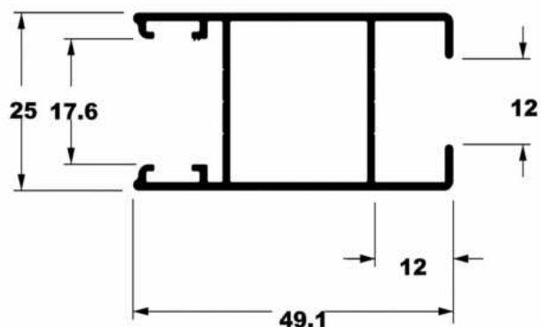
SU-057 0,631 Kg/m
