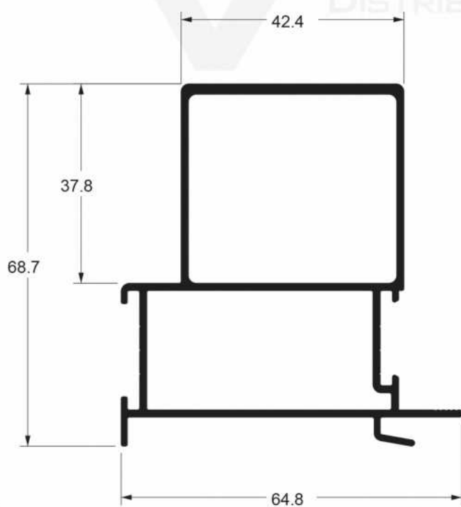
SU-289 1,217 Kg/m
