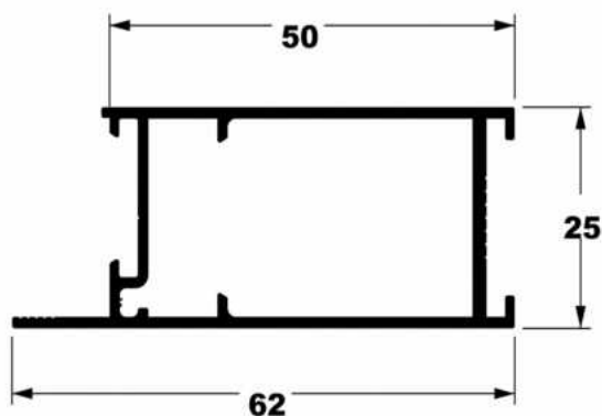
SU-276 0,169 Kg/m
