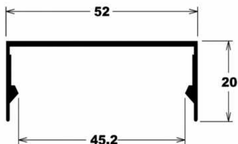
U-877 0,350 Kg/m
