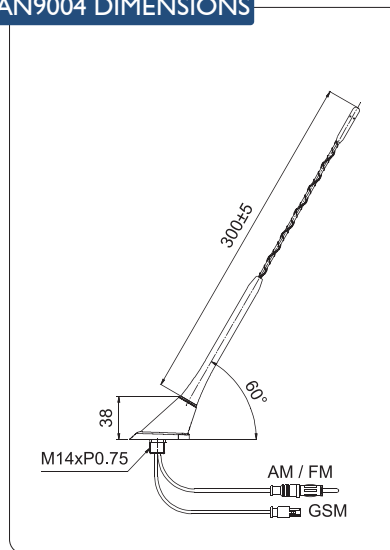
AN9004 DIMENSIONS
