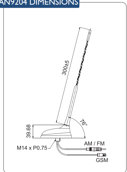
AN9204 DIMENSIONS
