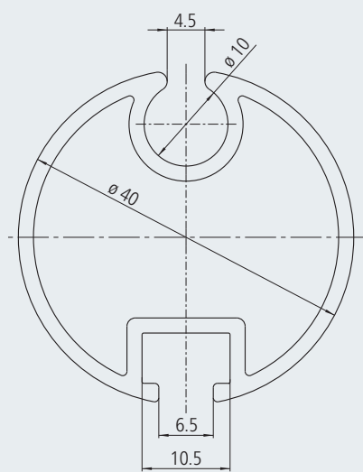
Doorsnede uitvalprofiel
